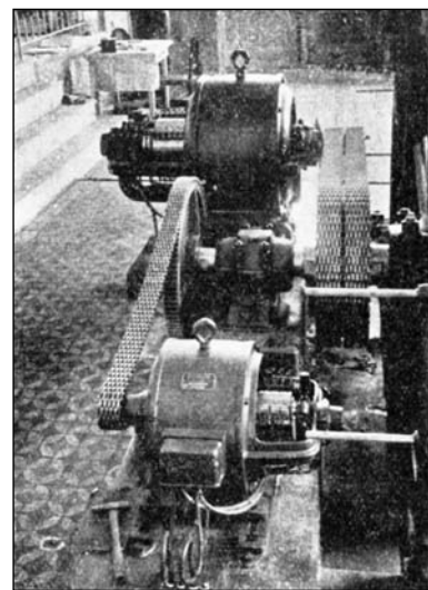
□ Hlavní a vedlejší dynamo
